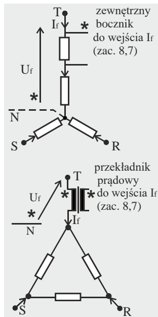
Rys. 1). Opis zacisków podłączeniowych
