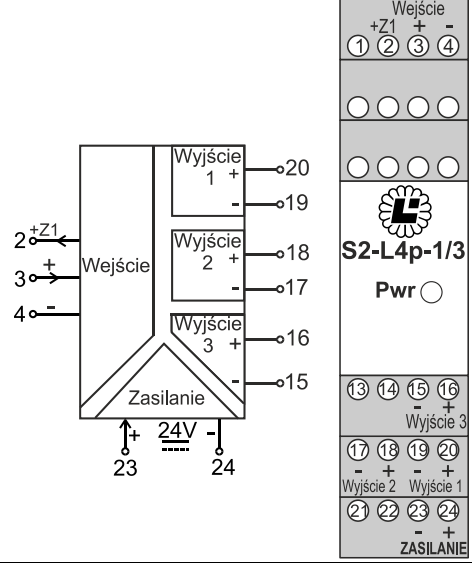
Rys.3 Opis zacisków powielacza trzutorowego S2-L4P-1/3-(R/R-R-R)
