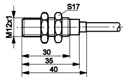
Czoło wbudowane
