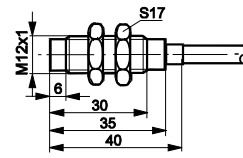
Czoło niewbudowane
