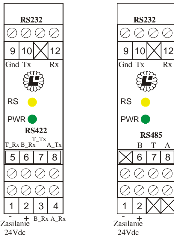
RYS. 1 Opis zacisków podłączeniowych
